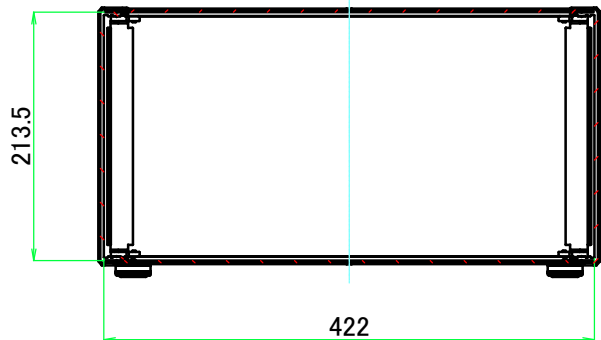
A-A ( 1 : 6.5 )
