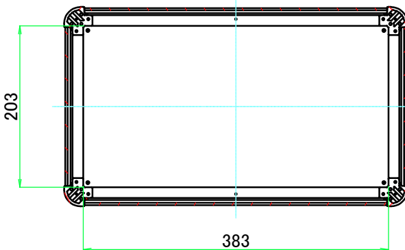
C-C ( 1 : 6.5 )
